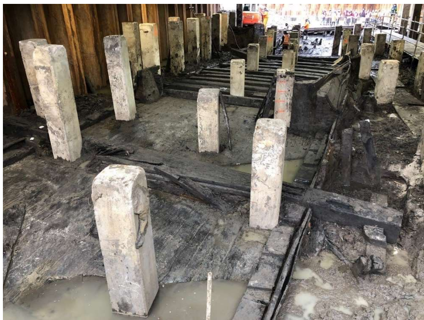
De betonnen palen van het nieuwe gemaal gaan dwars door de vroegere eikenhouten sluisvloer. (Foto Henri Willig).
